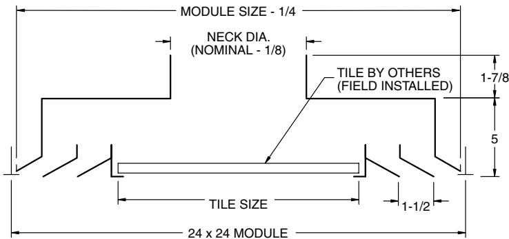
Model TML - Lay-In T-Bar
