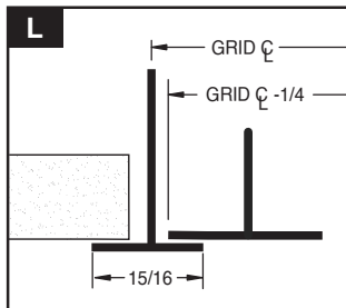
LAY-IN T-BAR (L)
